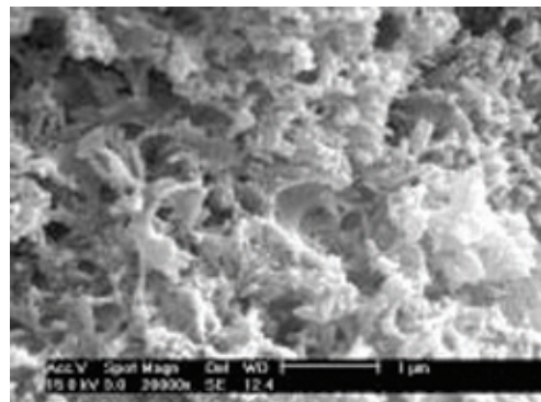
Микрофотография цементного раствора полученного при смешивании Keracolor FF и Fugolastic . Обратите внимание на более компактную структуру, из-за наличия полимеров в пустотах.
