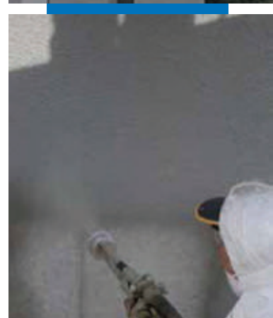
Нанесение Mapelastic на виадук путем распыления
